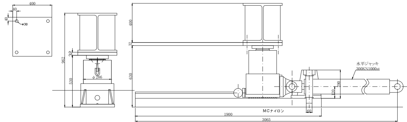
ジャッキヘッドプレート詳細
